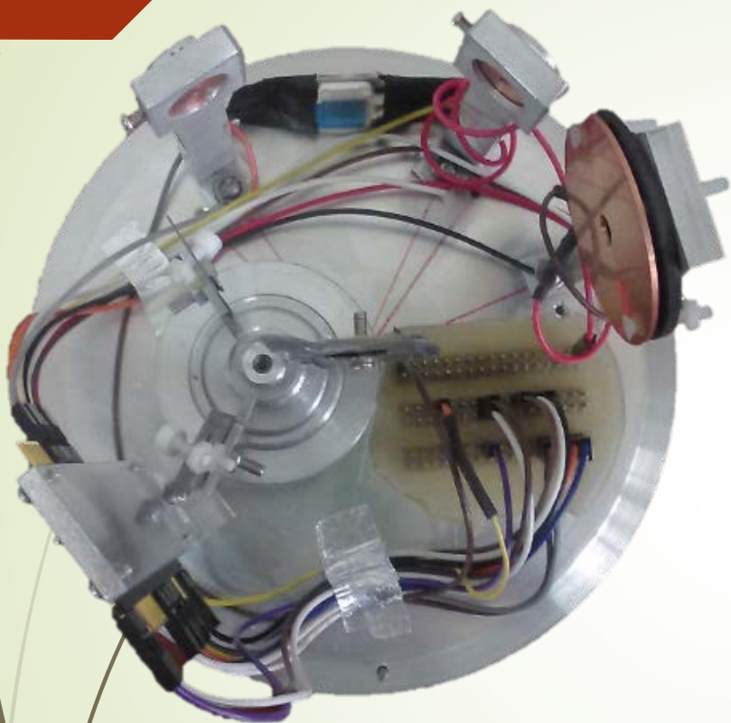
靶室实物图
